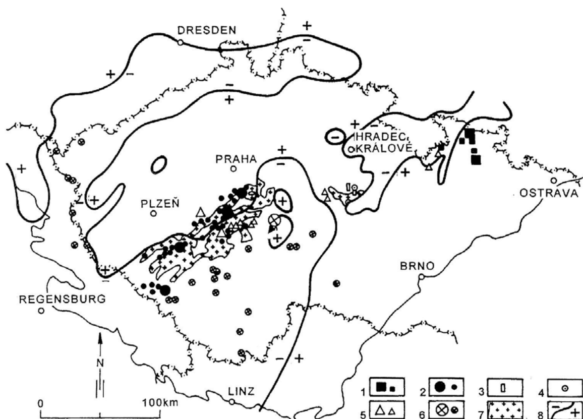
Obr. 17. Ložiska a výskyty zlata a rud antimonu v Českém masívu (podle Bernarda 1991): 1 – stratiformní ložiska a výskyty zlata v Jeseníkách, 2 – žilná ložiska a výskyty starovariské Au-mineralizace (asociace s-au ), 3 – aluviální výskyty zlata na Chrudimsku, 4 – výskyty rudních žil Pb-Zn se zvýšeným obsahem zlata, 5 – žilná ložiska a výskyty rud Sb (asociace sb ), 6 – žilná ložiska a výskyty středně variské Au-mineralizace (asociace au ), 7 – starovariské tonality a granodiority, 8 – rozhraní pozitivních a negativních regionálních gravimetrických anomálií (mGal).
