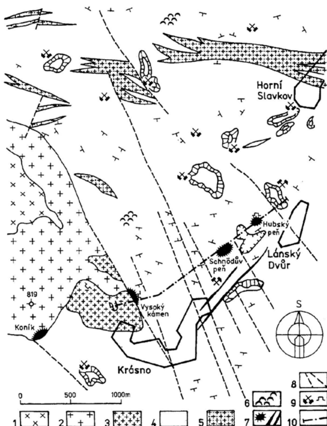
Obr. 18. Schematická mapa rudních ložisek v okolí Horního Slavkova (podle Jarchovského 1974): 1 – porfyrická jemnozrná žula, 2 – lithná albitická žula, 3 – aplity, 4 – krystalinikum, 5 – starší aplity, 6 – rýžoviště Sn, 7 – greiseny a rudní žíly Sn-W, 8 – poruchová tektonika, místy s křemennou výplní, 9 – šachty a štoly, 10 – osa těles greisenů.
