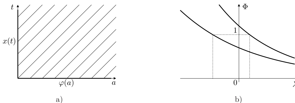
Obrázek 1.5: K řešení McKendrickovy-von Foersterovy rovnice. a) charakteristiky rovnice (1.98), b) možný průběh funkce \Phi , tj. pravé strany rovnice (1.113).
