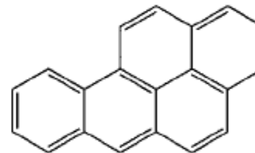
BaP
