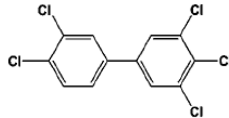
3,3',4,4',5-pentaCB
