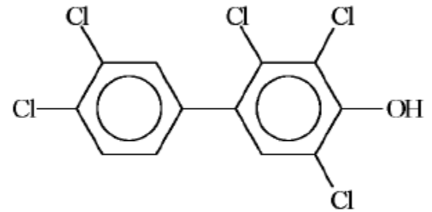
4-OH-PCB107
