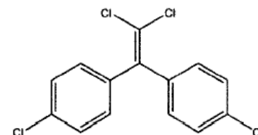
p,p' -DDE
