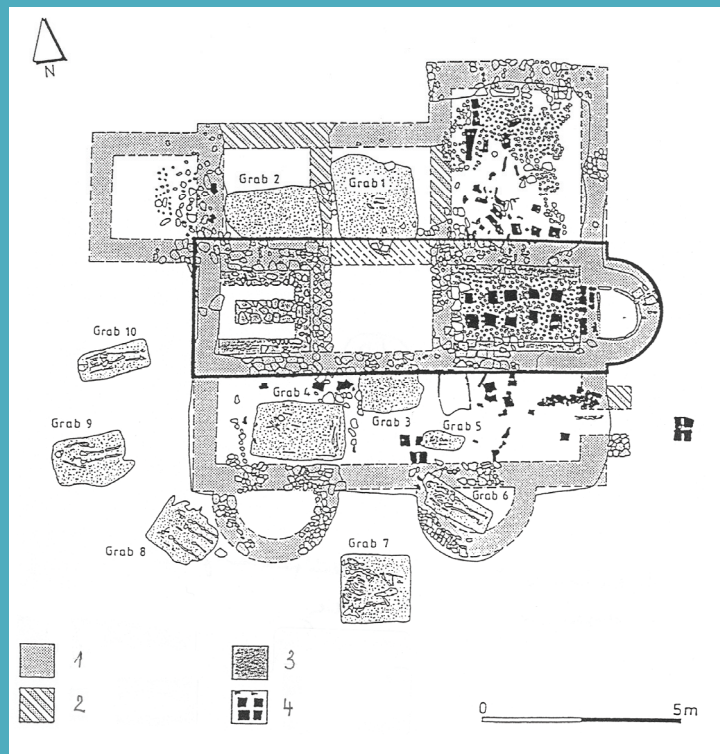
Pohřební kaple ze 7. století s deseti hroby postavená v Hartingu u Řezna v Bavorsku do zřícenin římských lázní. Legenda: 1 – zdivo a suť, 2 – doplnění, 3 – zděné přístavky, 4 – cihly.
