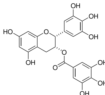
polyfenol v zeleném čaji
