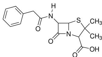
penicilin G
