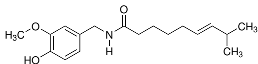
kapsaicin (co páří v paprice)
