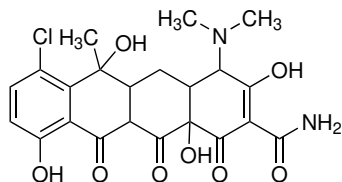
tetracyklin (anibiotikum)
