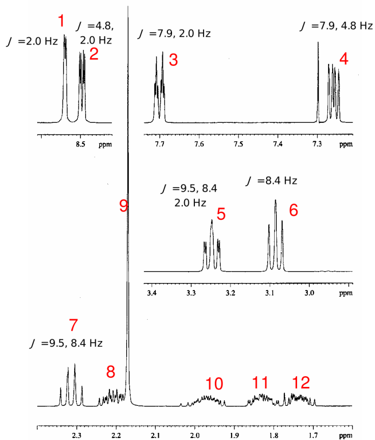
1 H NMR
