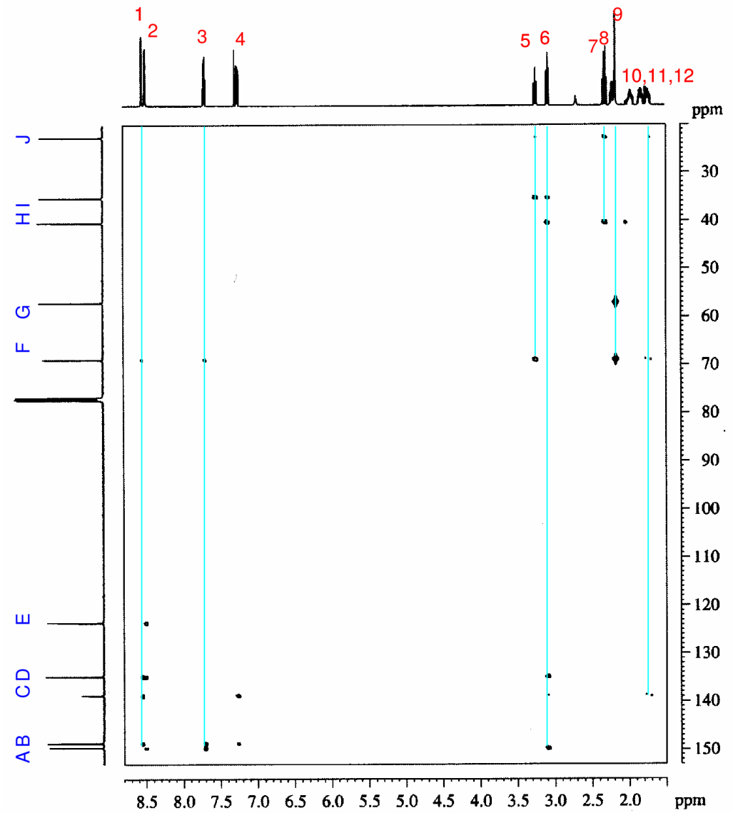
^{13}C, ^1H HMBC
