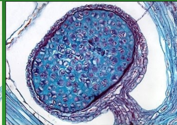
Lycopodium
