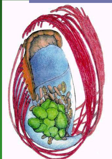
Phylloglossum drummondii
