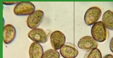
mikrospóry 20-40 µm
