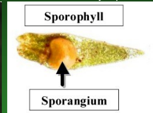
Lycopodium
