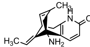
Huperzin A
