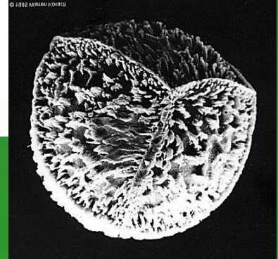
megaspóra
