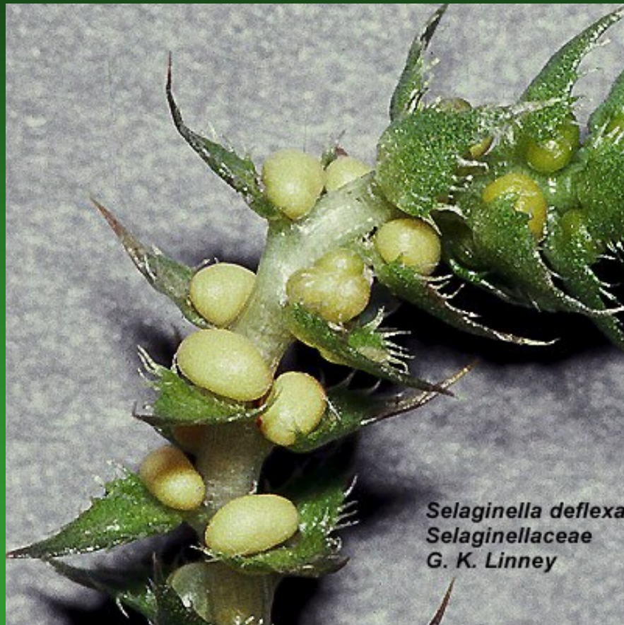
Selaginella
