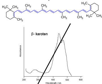
\beta -karoten
