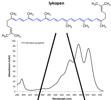
lykopen
