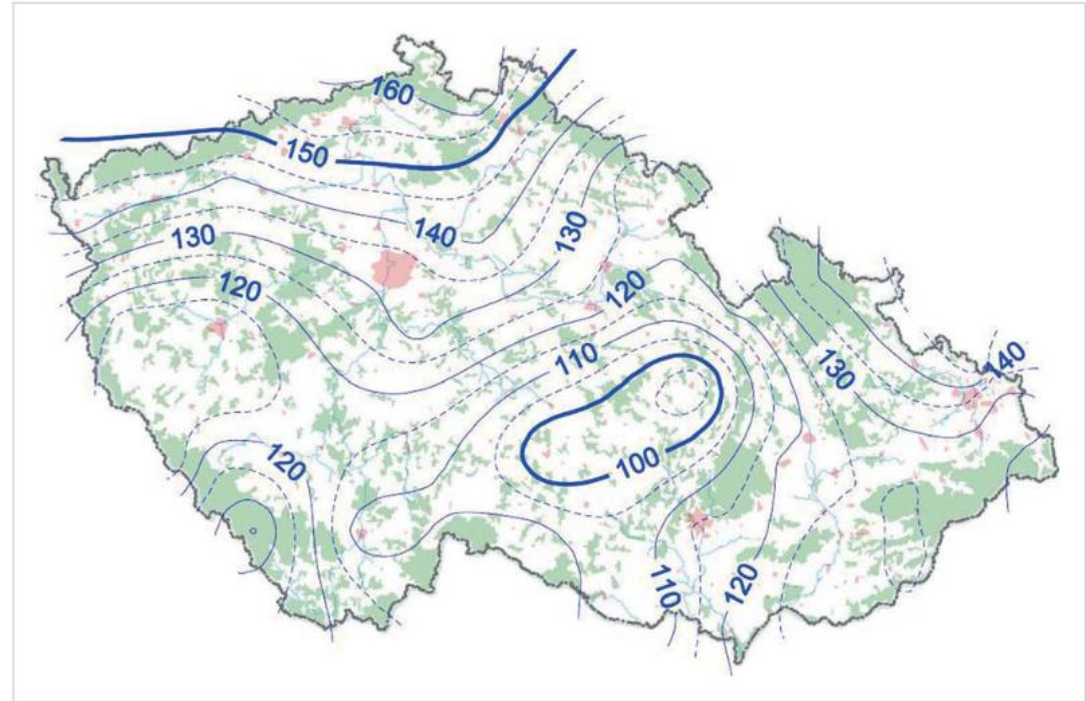
Obr. 8 Rozdíl výšek EVRS (EVRF2007) – Bpv na území ČR v milimetrech
