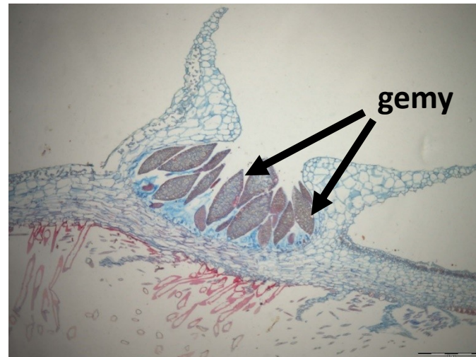
průřez thalidiem
