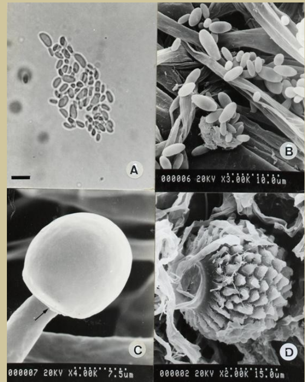
Mucor hiemalis
