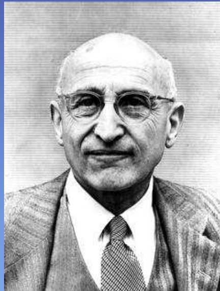
Beno Gutenberg (1889-1960)
