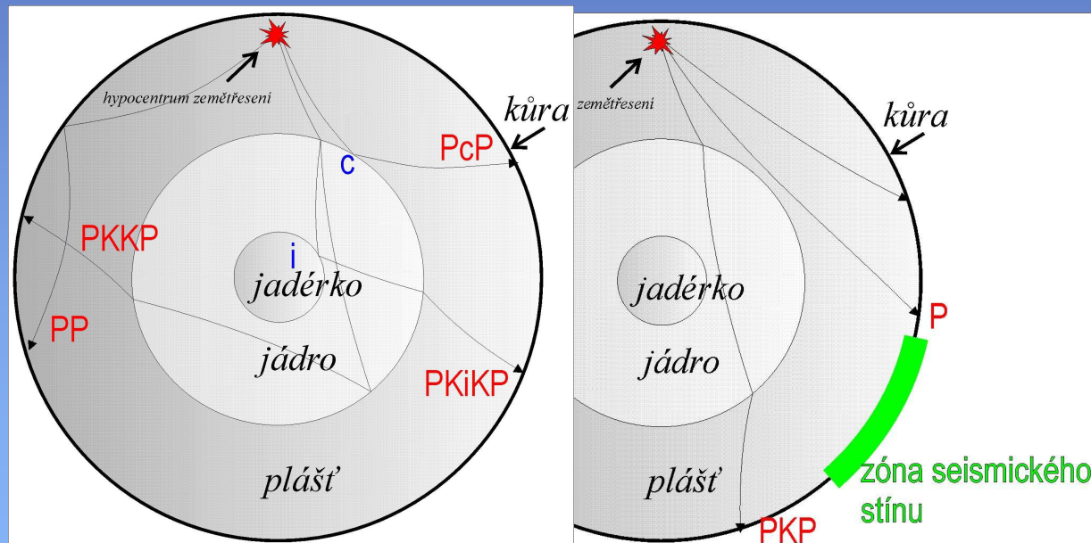
Inge Lehmannová (1888-1993)
