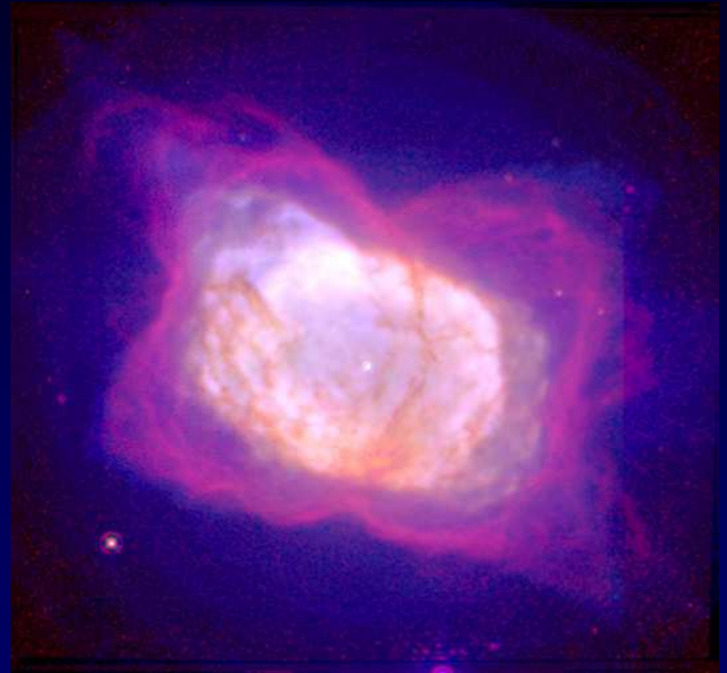
Planetární nebula NGC 7027
