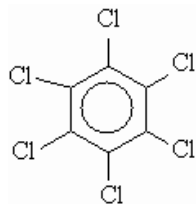
Hexachlorobenzene
