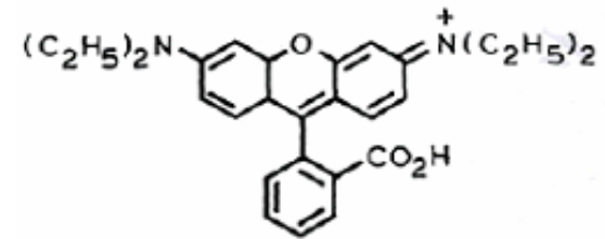
Rhodamine B
