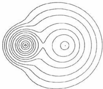
LiH
