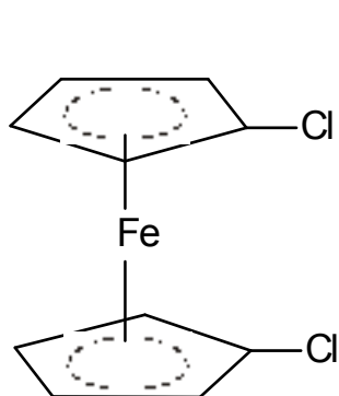
1,1'-dichloroferrocen
