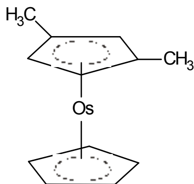
1,3-dimethylosmocen
