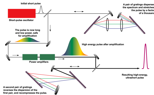
Obrázek 4: Laser s čerpováním
