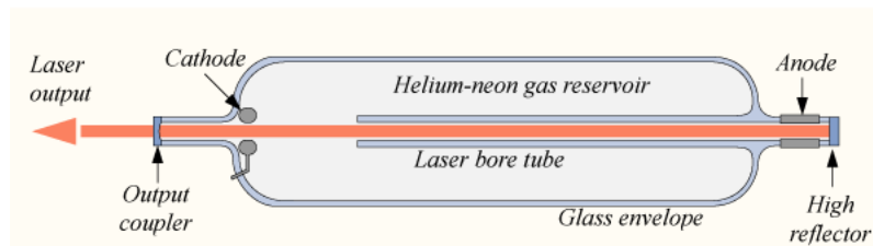
Obrázek 2: Základní schéma He-Ne laseru
