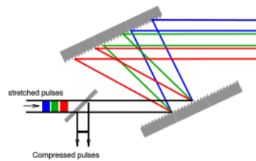
Obrázek 5: Rozkladné mřížky
