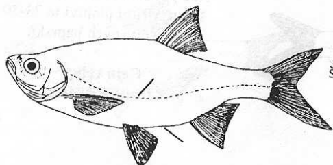
Perlín ostrobřichý ( Scardinius erythrophthalmus )
