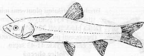
Amur bílý ( Ctenopharyngodon idella )
