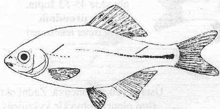
Hořavka duhová ( Rhodeus sericeus )
