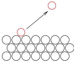
desorpce
