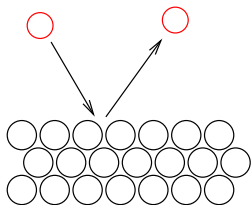
odraz molekuly
