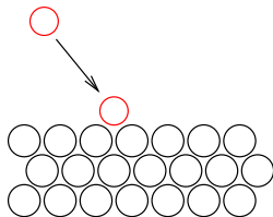
adsorpce
