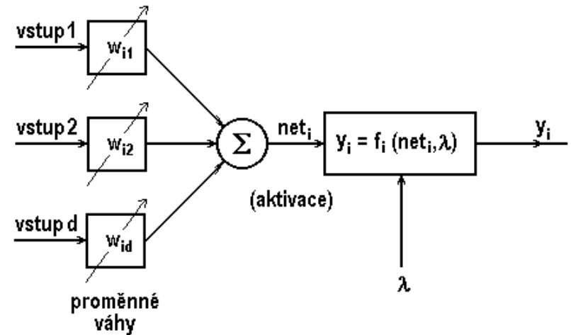
Výpočetní struktura umělého neuronu
