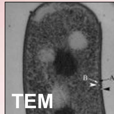
R. aetherivorans
