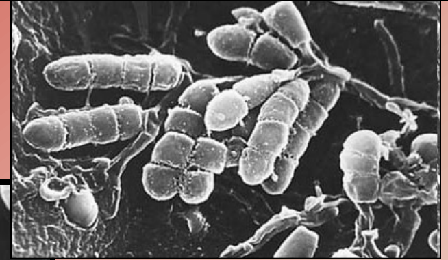
Microtetrastroma - tetrády
