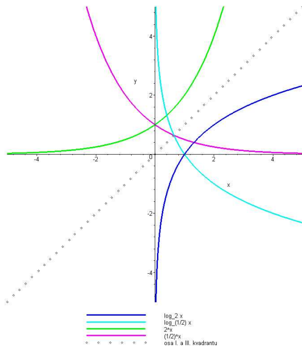
OBRÁZEK 12. Logaritmičké a exponenciální funkce.
