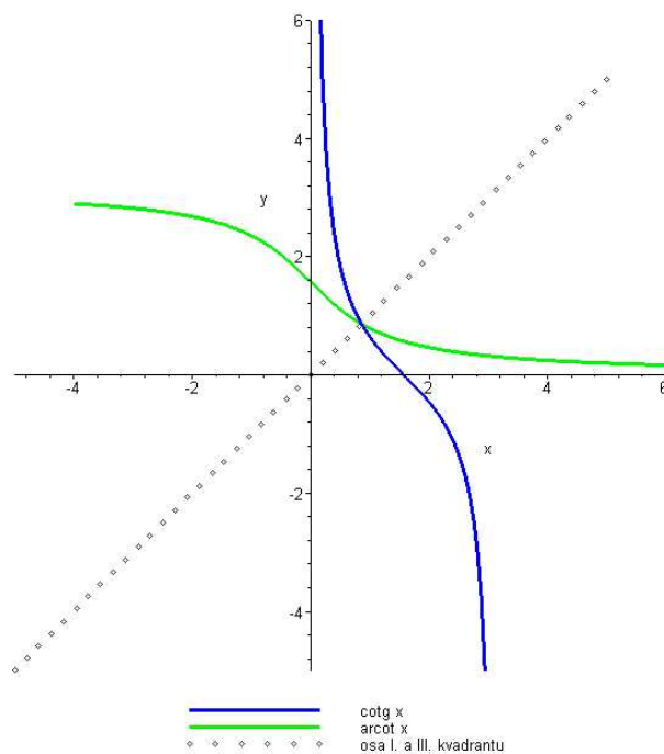
OBRÁZEK 10. Funkce arkuskotangens.
