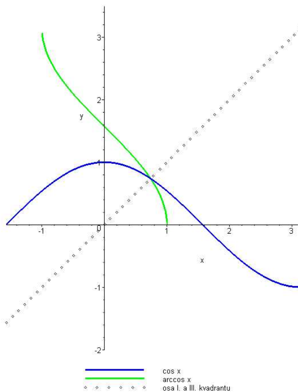
OBRÁZEK 8. Funkce arkuskosinus.
