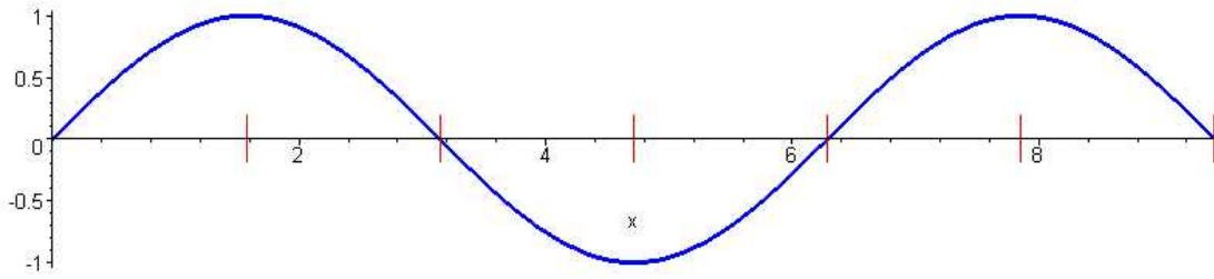
OBRÁZEK 1. Funkce sinus.
