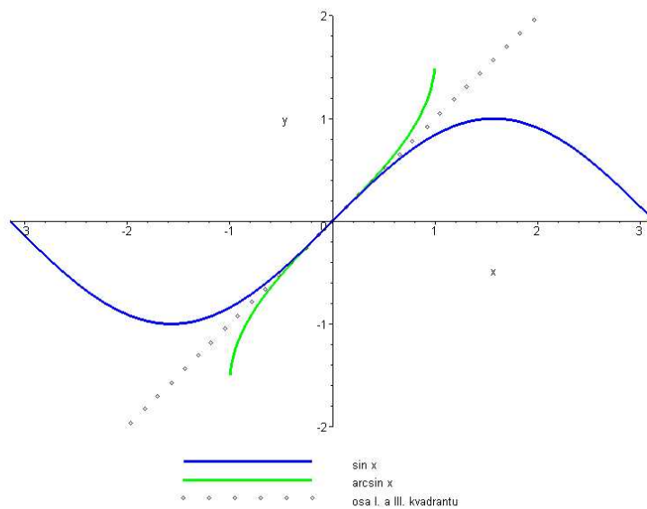
OBRÁZEK 7. Funkce arkussinus.
