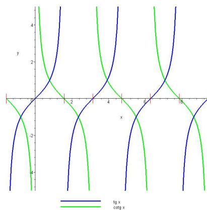
OBRÁZEK 6. Funkce tangens a kotangens.
