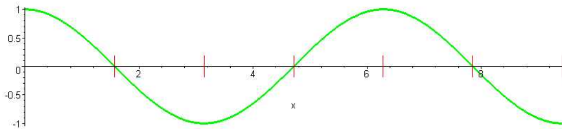
OBRÁZEK 2. Funkce kosinus.
