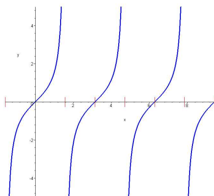
OBRÁZEK 4. Funkce tangens.
