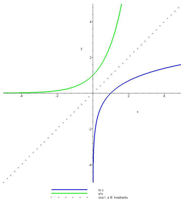
OBRÁZEK 11. Funkce e^x , \ln x .
