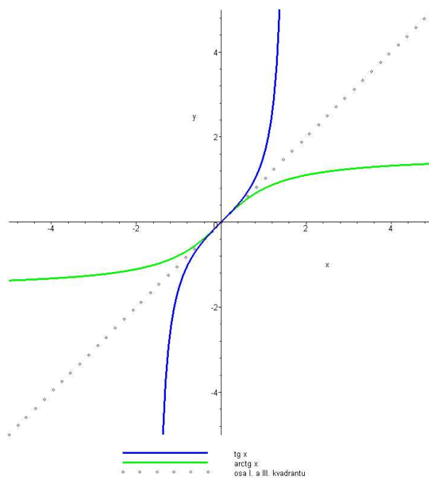
OBRÁZEK 9. Funkce arkustangens.
