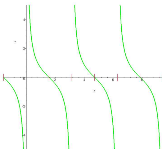
OBRÁZEK 5. Funkce kotangens.
