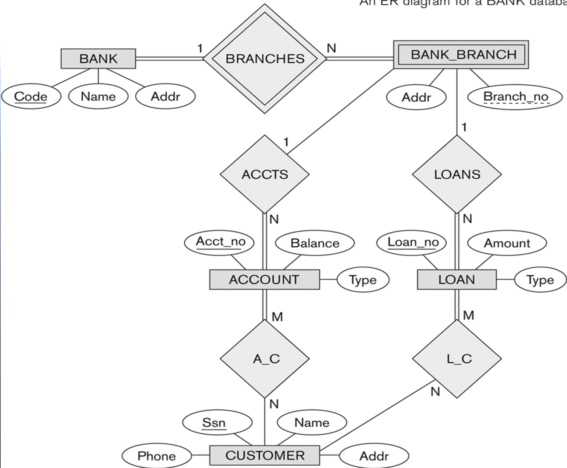
An ER diagram for a BANK database schema.
