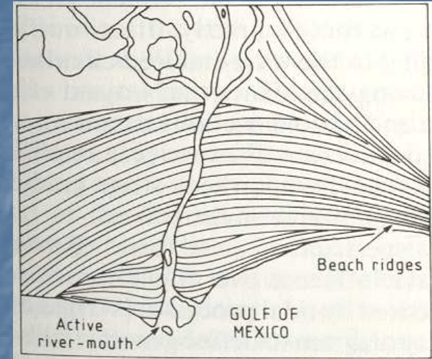
Lukovitá delta
