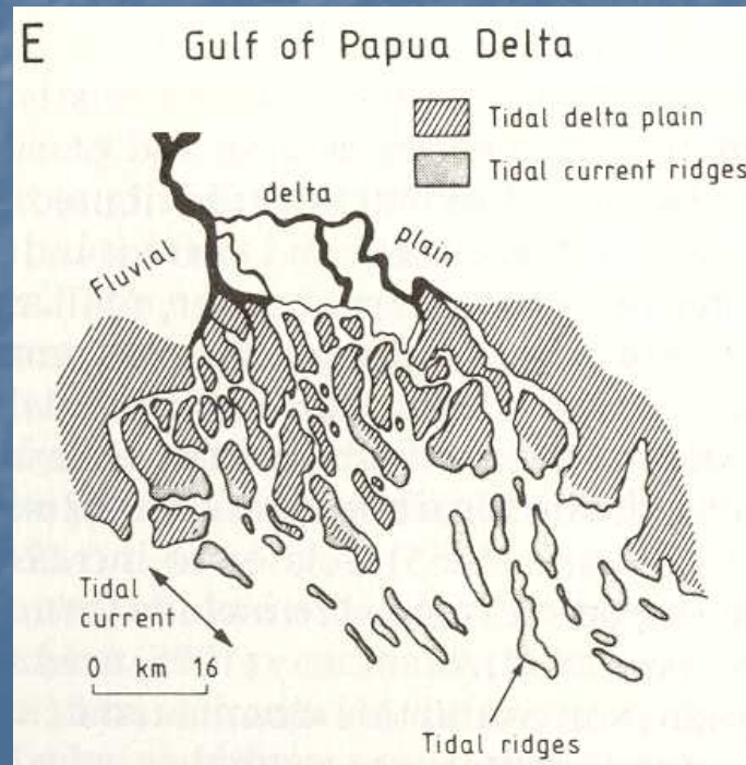
Odlivová delta
