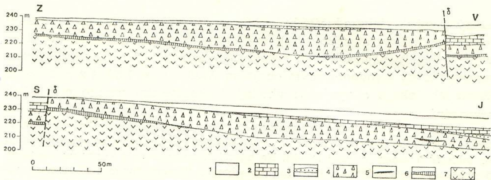
52. Geologický řez částí ložiska Lahošť—Jeníkov (podle J. Kohouta upravil J. Franče) 1 — sraše, srašové a svahové hlíny; 2—6 křída (svrch. turon); 2 — slíny, slínovce, jíly, jílovce; 3 — nadložní slepence; 4 — křemenec; 5 — jílovce se zuhelnatělými rostlinnými zbytky; 6 — slepence; 7 — křemenný porfyr (perm).
