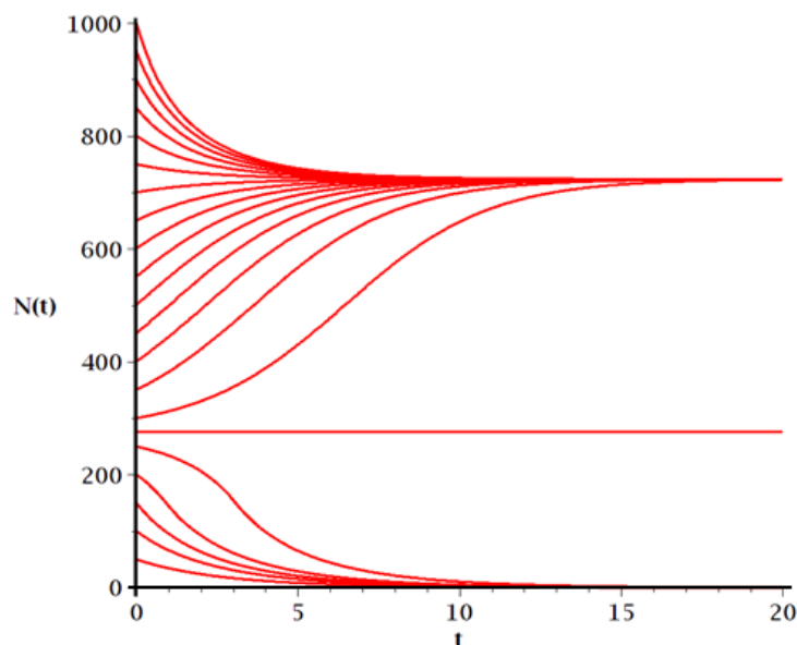
Obrázek 3.25: Řešení modelu růstu populace pod tlakem nesespecializovaného predátora v případě 2. c)
