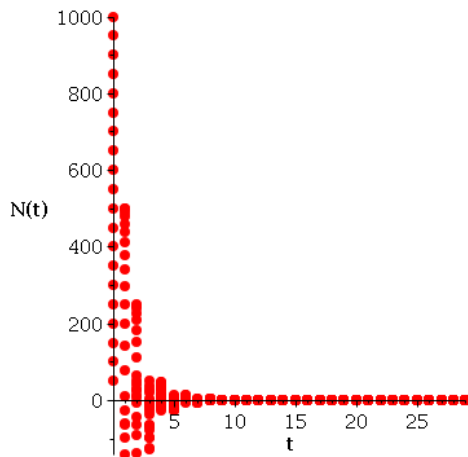
Obrázek 3.27: Řešení modelu růstu populace pod tlakem nespécializovaného predátora v diskretní podobě případu 1. a)
