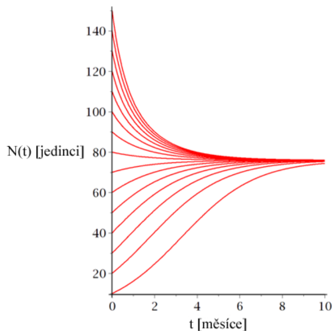
Obrázek 3.10: Vykreslení závislosti řešení na počáteční velikosti populace
