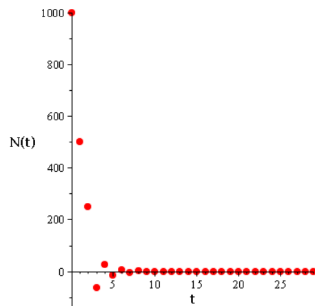
Obrázek 3.27: Řešení modelu růstu populace pod tlakem nespécializovaného predátora v diskretní podobě případu 1. a)
