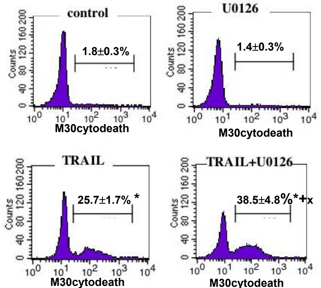
Štěpení CK18 (M30cytodeath, FCM)
