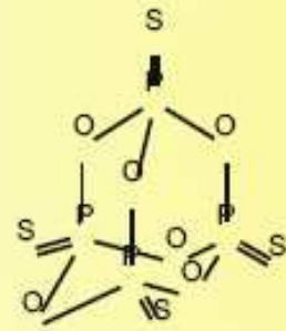
P_4O_6S_4
