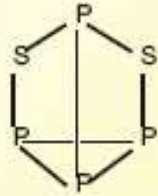
P_4S_2
