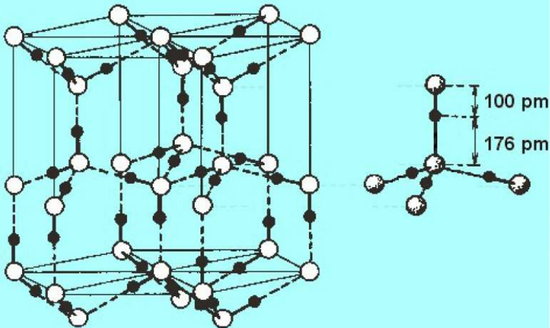
Struktura ledu I h
