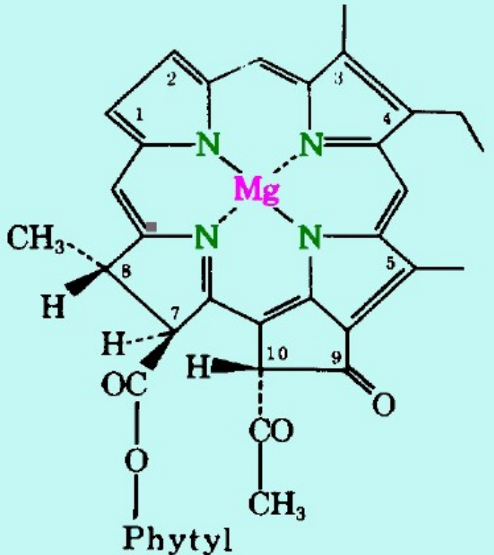
Chlorofyl
