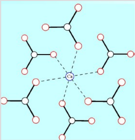
kalцит
