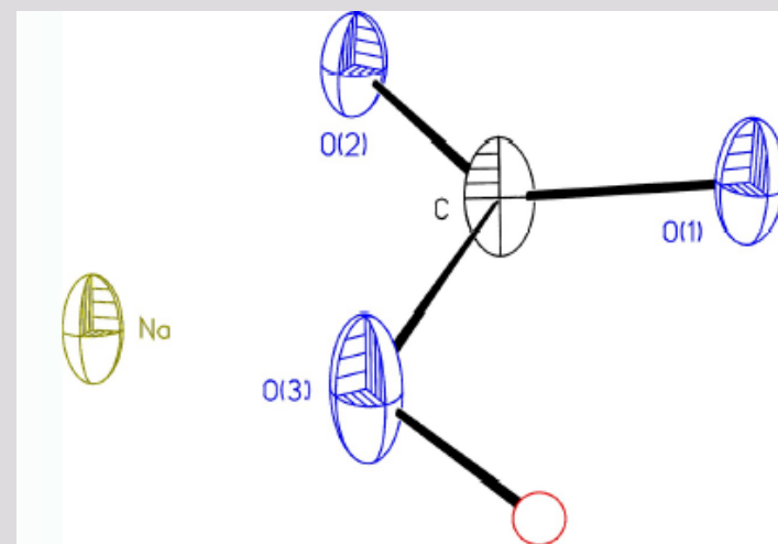
struktura \text{NaHCO}_3
