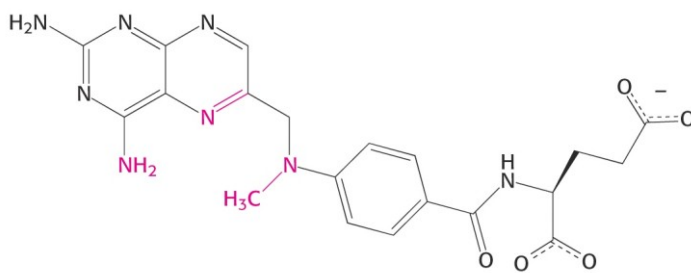
Methotrexate
