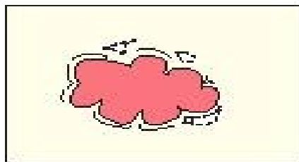
In-situ melting
