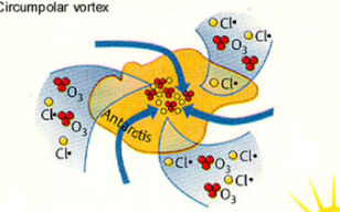
Circumpolar vortex
