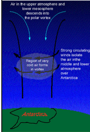
Circumpolar vortex
