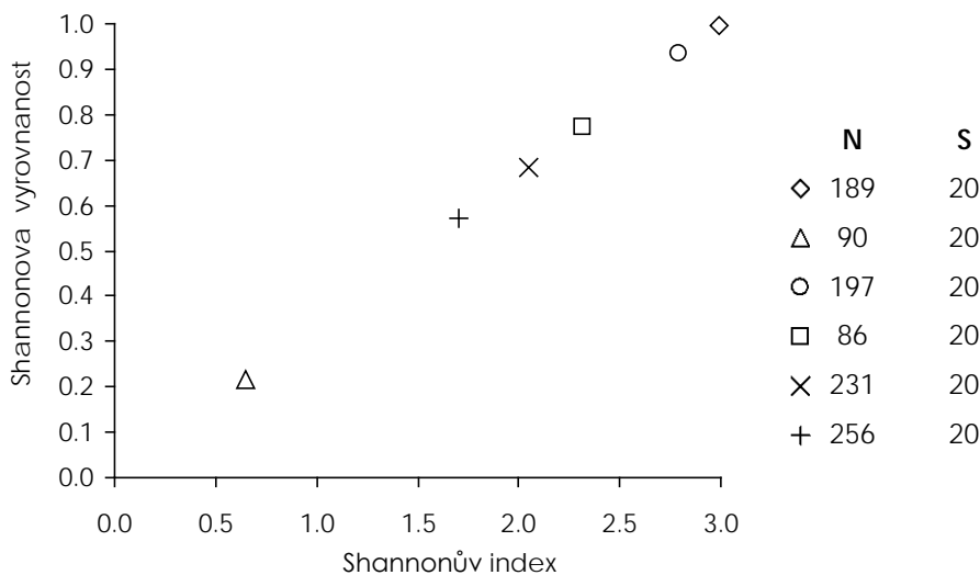
Obr. 4.4 Vztah Shannonova-Weaverova indexu a jeho vyrovnanosti při různém tvaru křivky společenstva Brillouinův index [31, 34]
