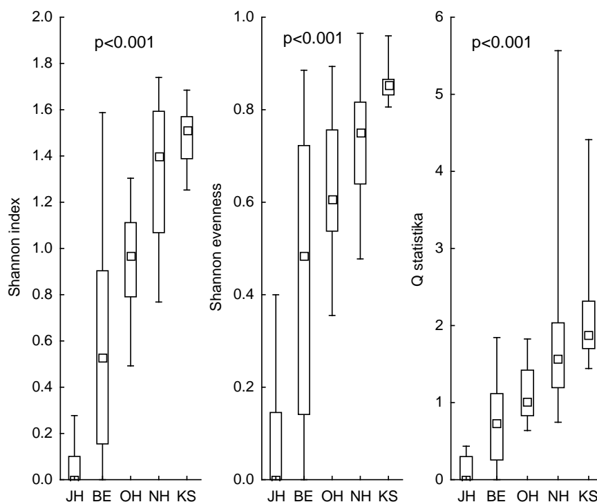
Obr. 12.4 Biodiverzitní indexy v jednotlivých oblastech (popsány mediánem, kvartily a 5-95ti percentilovým rozsahem); statistická významnost hodnocena Kruskalovým-Wallisovým testem.
