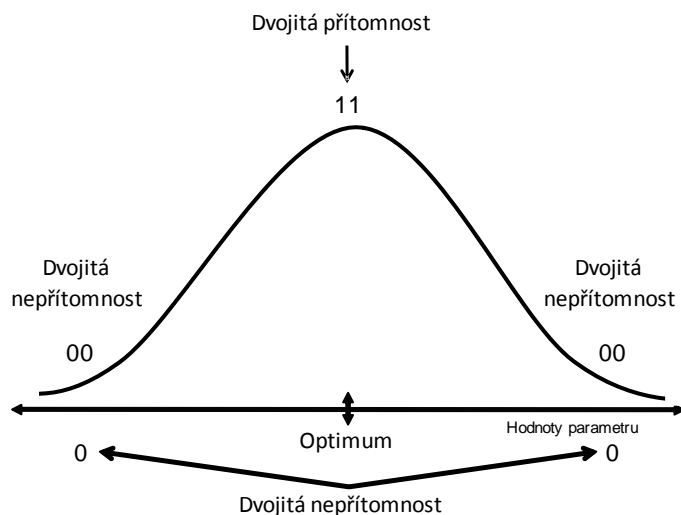
Obr. 8.1 Problém dvojité nepřítomnosti. Dvojitá nepřítomnost není stejná jako dvojitá přítomnost.
