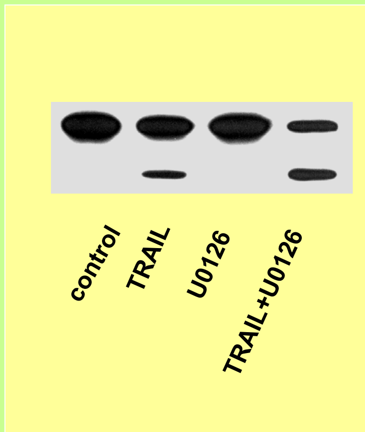
Štěpení PARP
