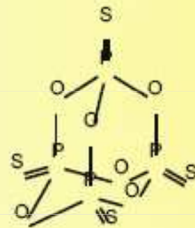
P_4O_6S_4
