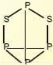
P_4S_2
