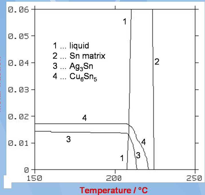
Obr. 15: Predikované fázové složení v závislosti na teplotě pro Sn-Bi-Cu-Ag.
