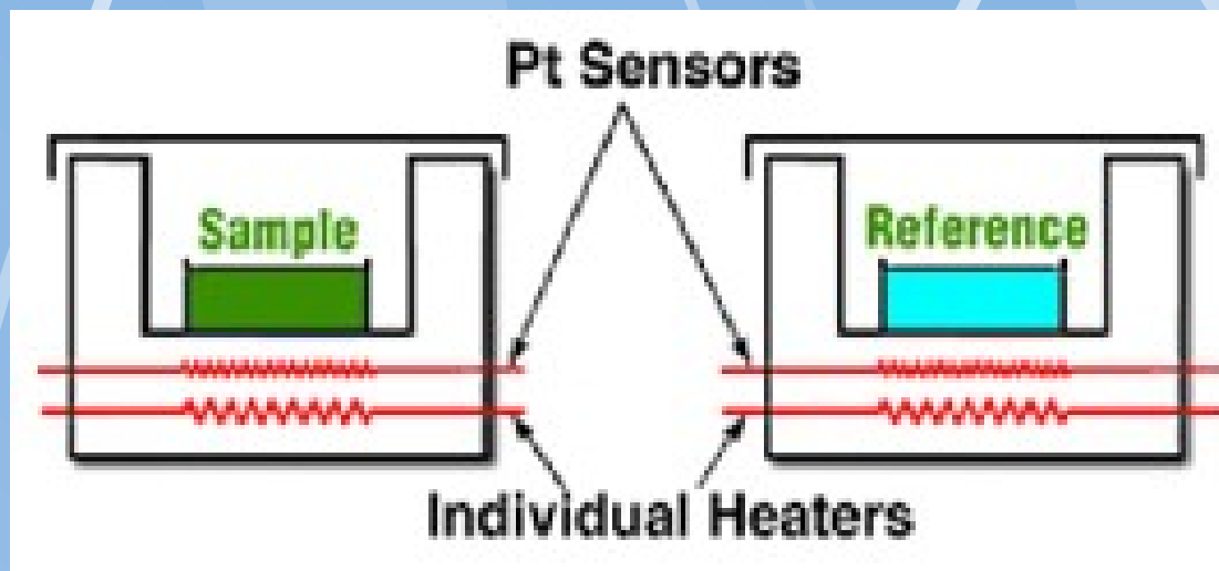
Obr. 7: Schéma kompenzační DSC
