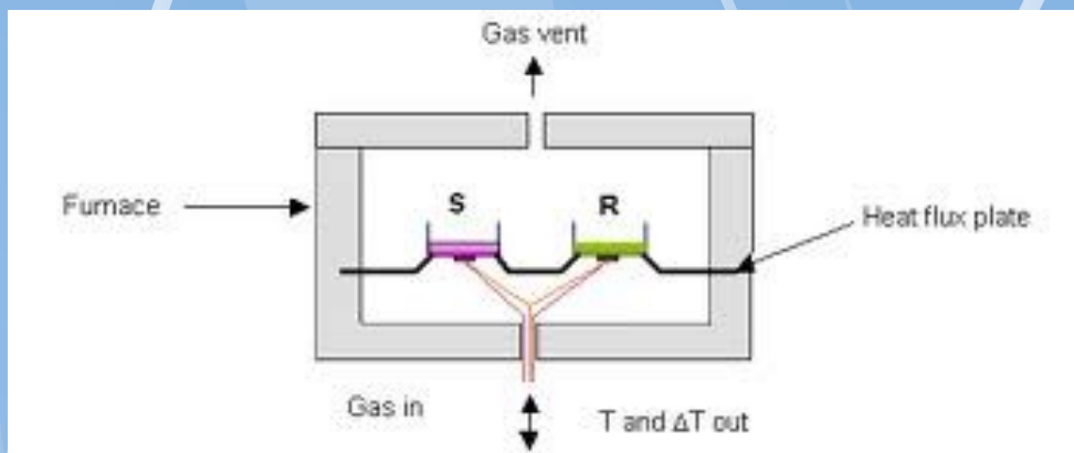
Obr. 9: Schéma DSC
