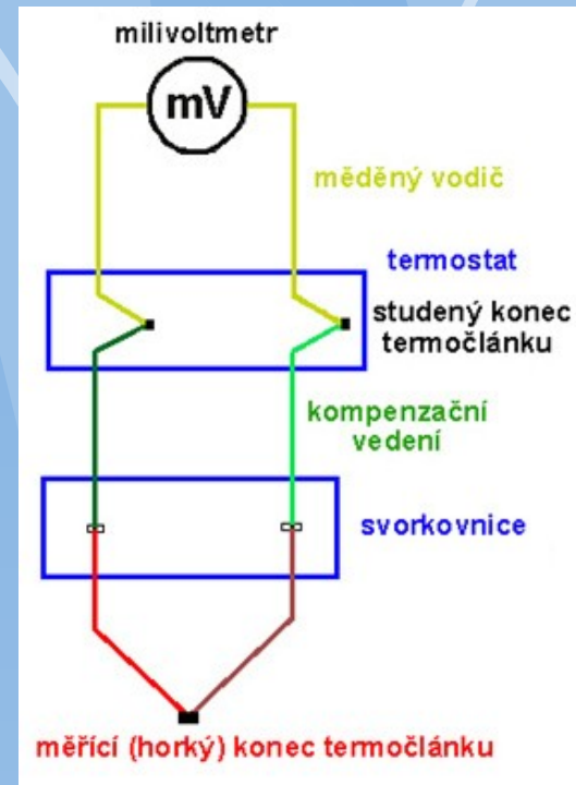
Obr.11: Schéma zapojení termočlátku
