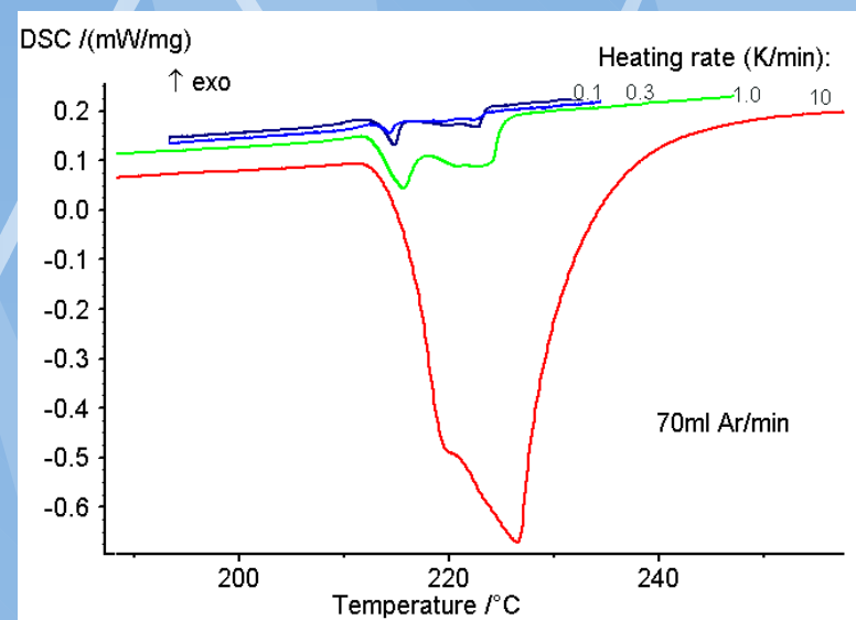
Obr. 17: Reálné DSC signály pro vbranou slitinu Sn-Bi-Cu-Ag za různé rychlosti ohřevu (extrapolace na rovnovážný stav).
