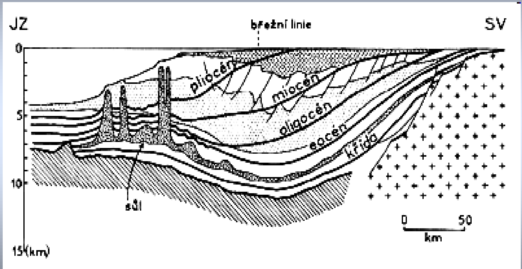
Řez deltou řeky Niger (Nigérie) znázorňující solné diapiry (pně), www.geology.cz
