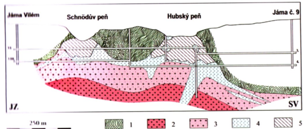
Geologický řez ložiskem Krásno-Horní Slavkov. 1 - migmatizované biotitické ruly, 2 - žuly, 3 - kaolinizované a sericitizované žuly, 4 - greiseny, 5 - vytěžené a zavalené partie pňů. Zpracoval: J. Tvrď
