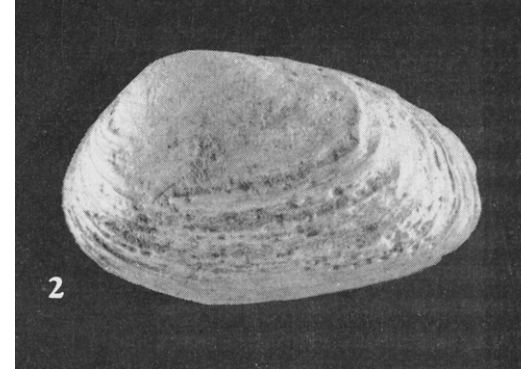
Rzhakia socialis socialis (Rzhak) Maršovice-Jezeřany, rzhakiové vr., ottnang (Foto Steininger et al. 1973)
