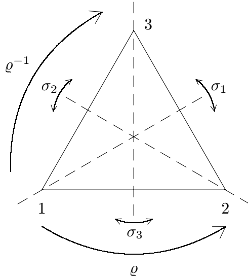
Obr. 0.1. Symetrie rovnostranného trojuholníka
