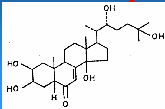
Ecdysone
