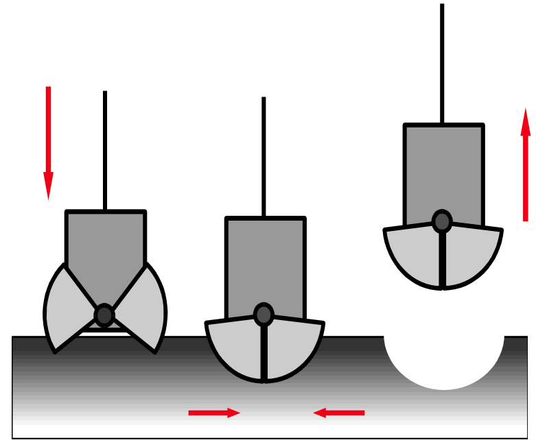
Grab probe
