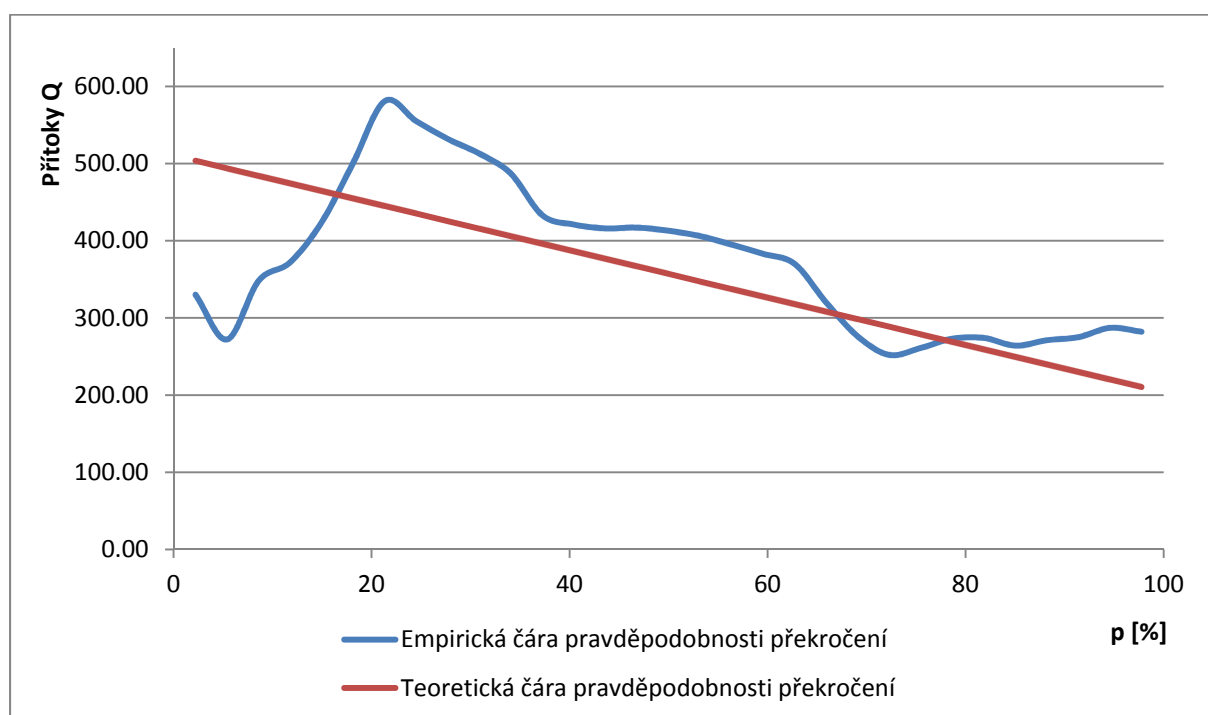
Obř. 2: Empirická a teoretická čára pravděpodobnosti překročení přítoku na řece Vltavě ve stanici Praha Chuchle v měsíci březnu pro rok 2009
