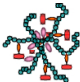
micelární systém
