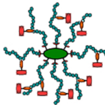
hypervětvený konjugát
