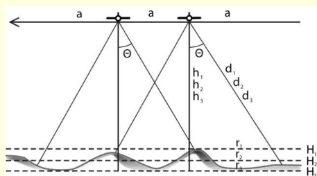
Obr. 1. Parametry leteckého laserového skenování.
