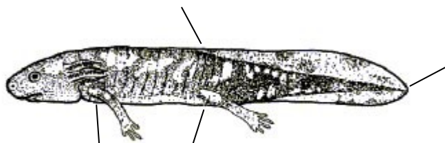
Obr. 4. Mlok skvrnitý
