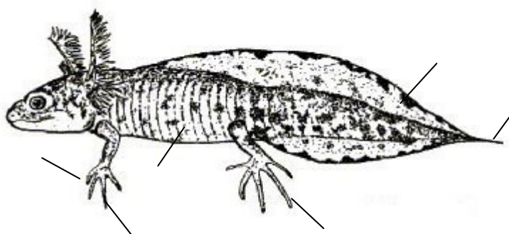
Obr. 5. Čolek velký
