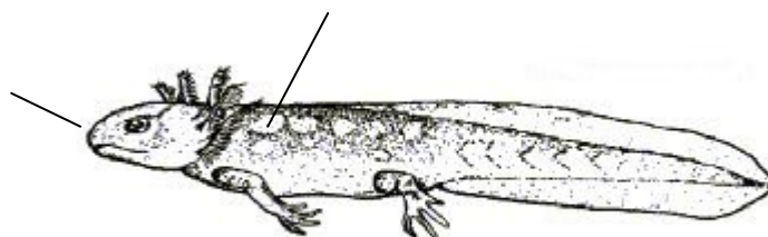
Obr. 9. Čolek karpatský
