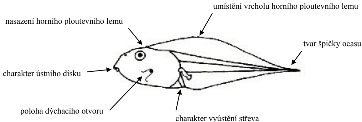
Obr. 2. Pulec
