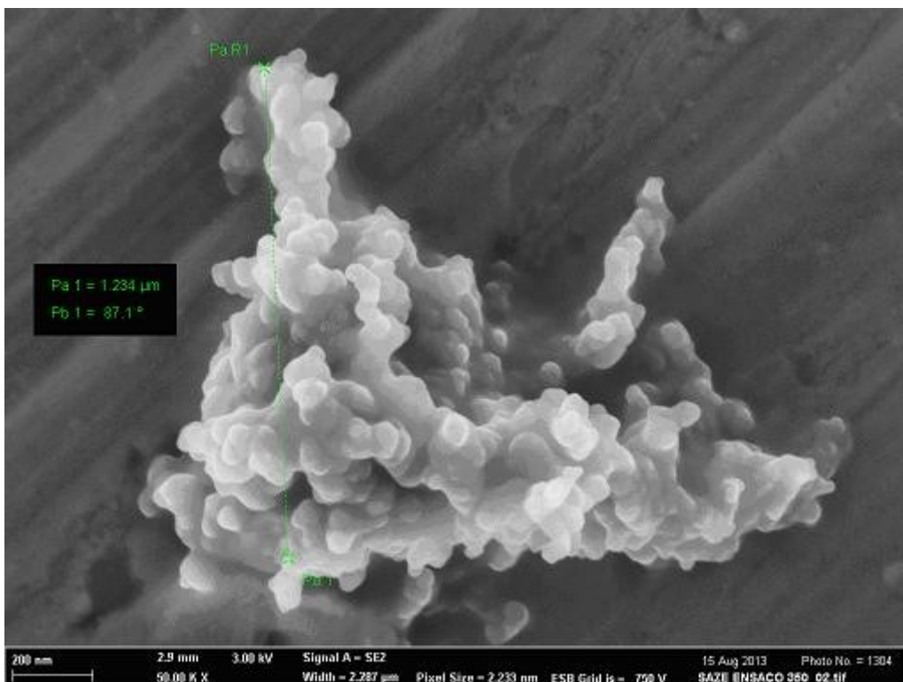
Morfologie částic ELEKTROVODIVÝCH sazí; zvětšení 50 000
