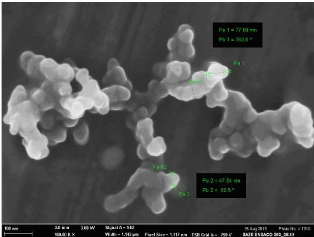
Morfologie částic ELEKTROVODIVÝCH sazí; zvětšení 100 000
